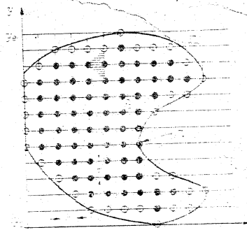
Implicit method ○ 境界点 ● 内点
