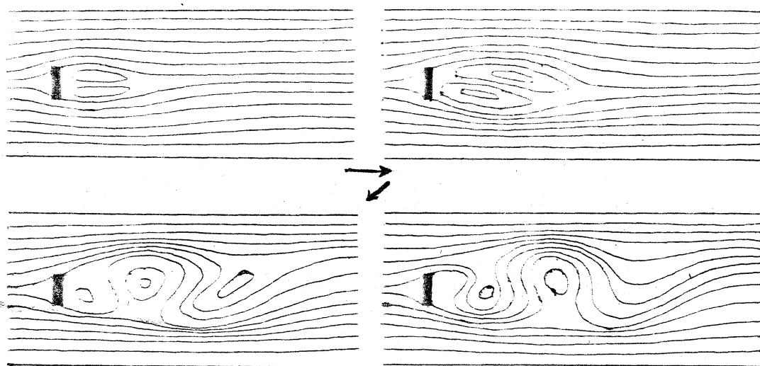
非対称攪乱から Kármán 渦列が形成される (Fromm, 1963)
