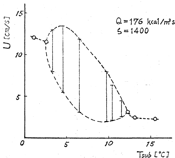
第8図 加熱部入口流速の振中
