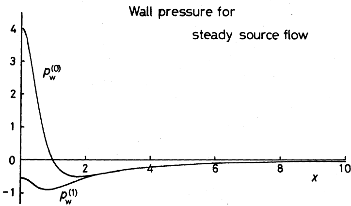
図5. 定常流に対する壁面圧力分布.
