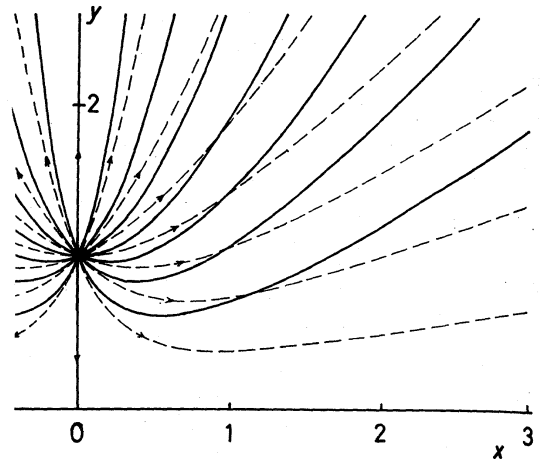
図2. 図1に対する定常 Stokes 流, および定常渦を流 (破線) の流線. ( \psi は等間隔)
