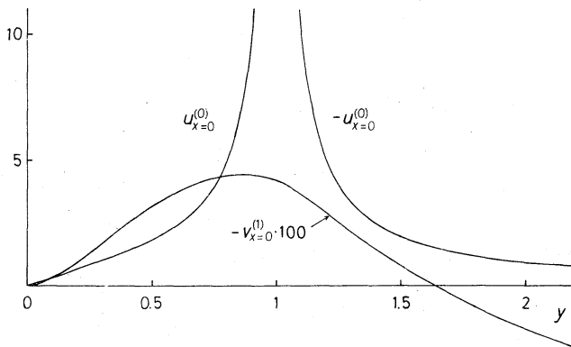
図11. 中心軸上の速度 分布. O(R) の補正項 は系統に100倍 [である [式(6.10), (6.11)参照].
