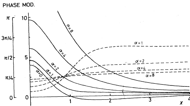
図8. 正弦的に強さの变化する点渦による壁面おり忘力。実線はその絶対値、破線は位相角を表わす。 \alpha=0 は定常解そのものを示す [式(6.2)参照]。
