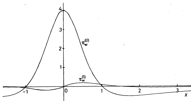
図9 定常流に対する壁面おり忘力分布 [式(6.6), (6.7)参照]。
