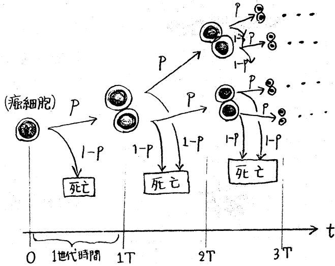
図 2.5. 癌細胞の増殖に関する分枝モデル 各癌細胞は分裂の直後から1世代時間 T を経過するまでに生存率 1-p で死亡(細胞死)し、もしも死亡しなかったなら、その都度2個の癌細胞に分裂して増殖する。
