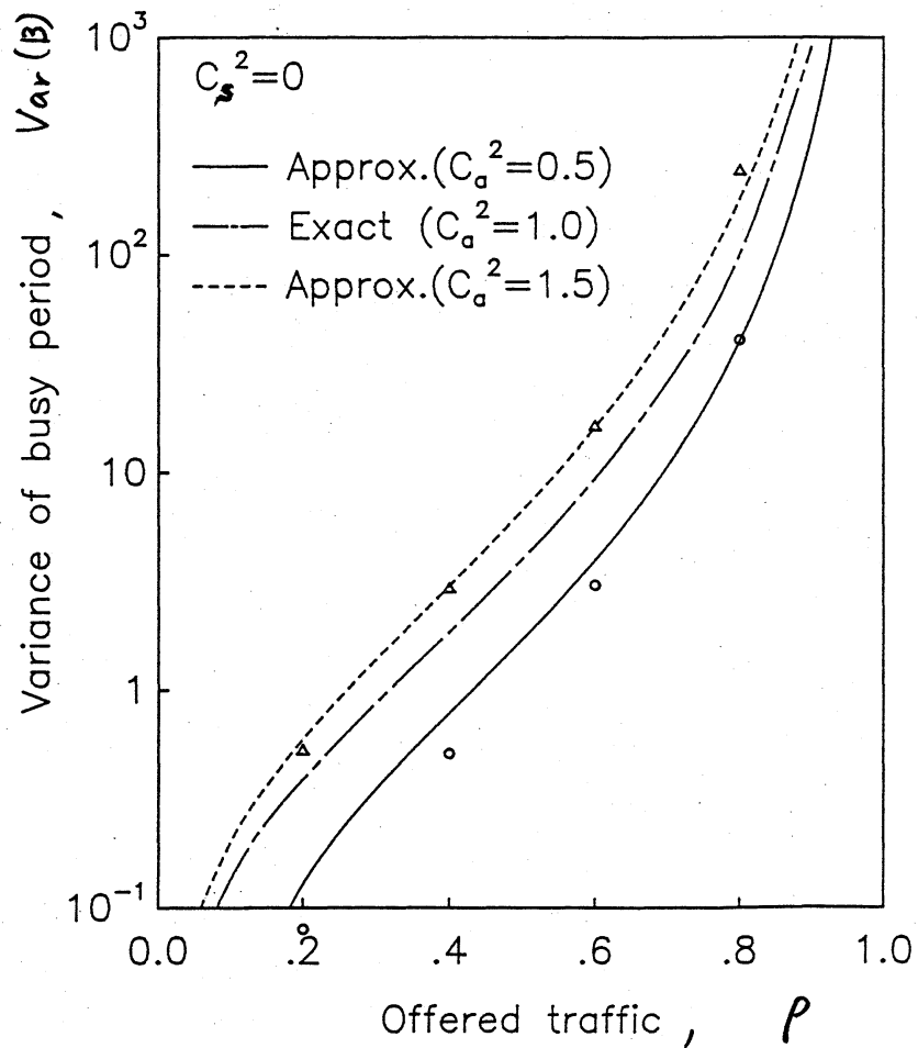
図4. 全稼働期間の分散 vs. \rho ( GI/p/1 )
