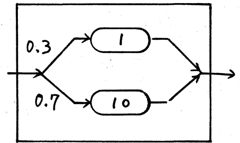
図2. 2-次超指数分布 (Ramaswamiの例 [18] )
