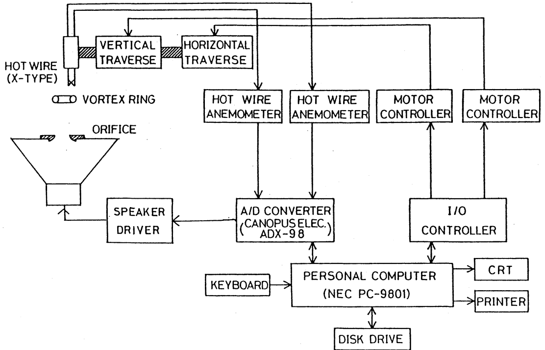
3 図 測定装置のブロックダイヤグラム
