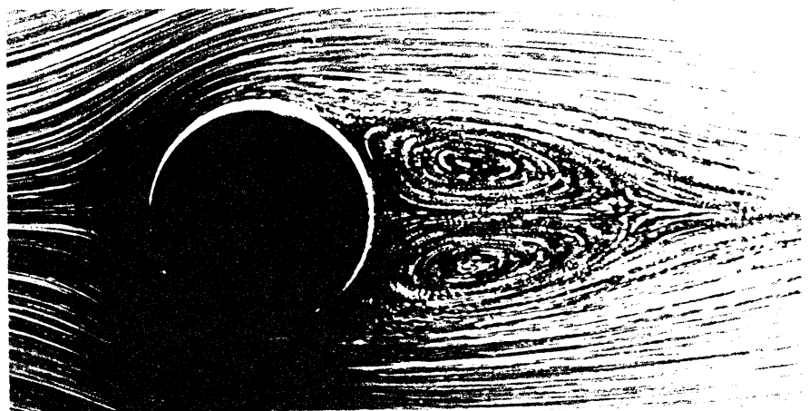
図 2 円柱まわりの流れ R=26
