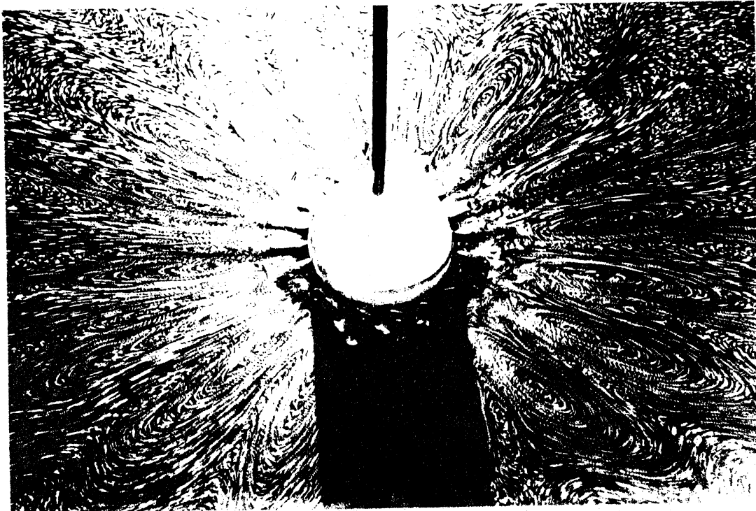
図 24 半没振動球まわりの水面波と水流 (球直径 3.8 cm, 振動数 30 Hz, 振幅 2.1 mm)
