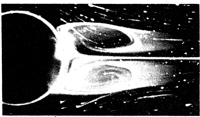
(b) 加速直後 R=149
