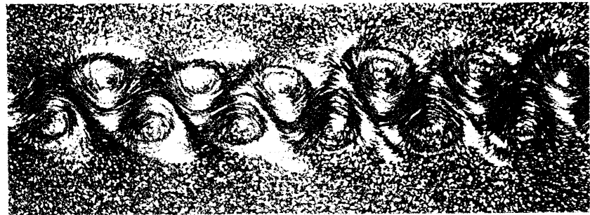
図12 迎角 0^\circ 平板の後流 R=15800
