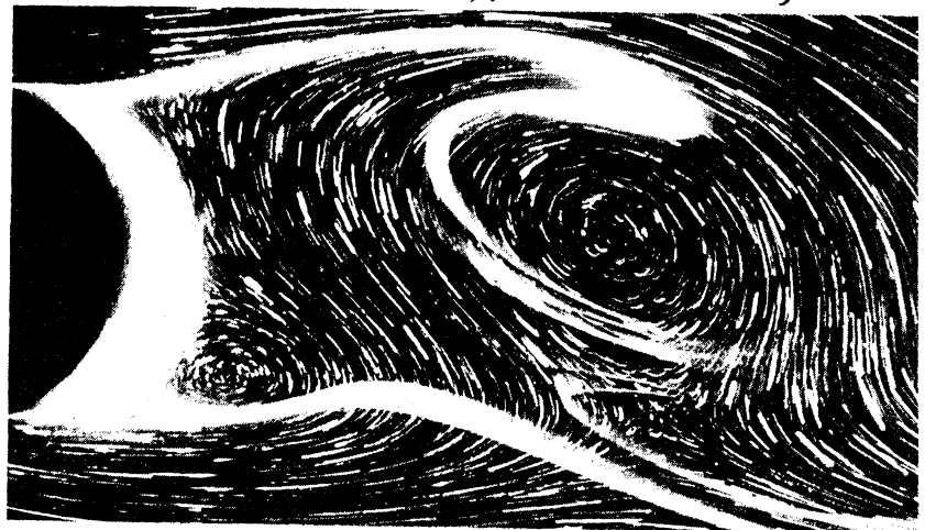
図11 円柱後流の流線と流脈
