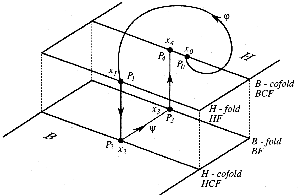
Fig. 9. Poincaré map T : BCF \rightarrow BCF ; x_0 \mapsto x_4 .
