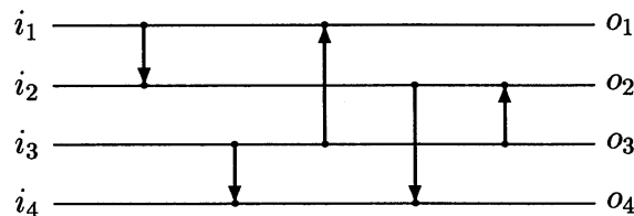
図 1: 比較器回路網の図示
