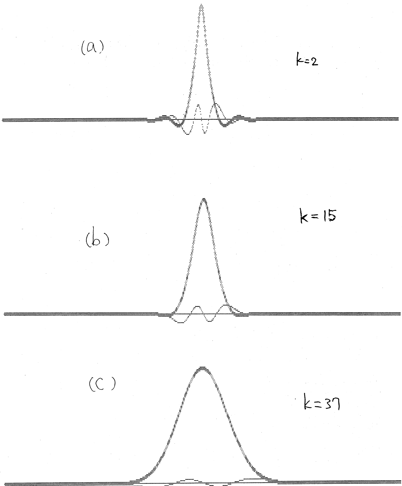
図 1 : |0\rangle_{F_k} の波動関数
