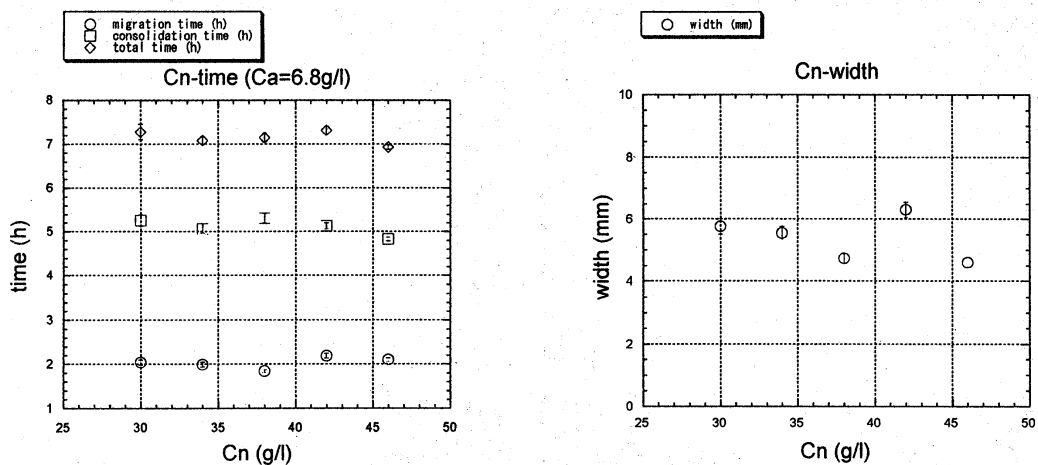
図 3 (a) migration time、consolidation time、cycle time の Cn 依存性
