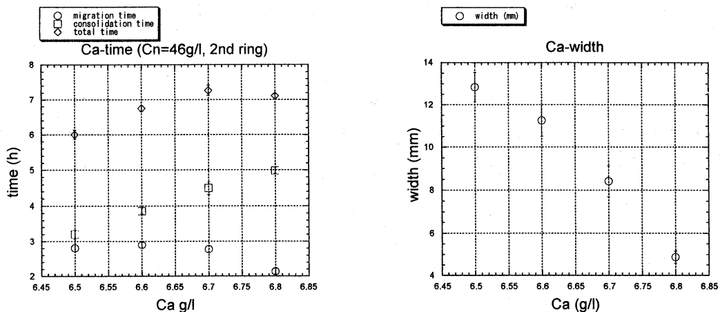
図 4 (a) migration time、consolidation time、cycle time の Ca 依存性
