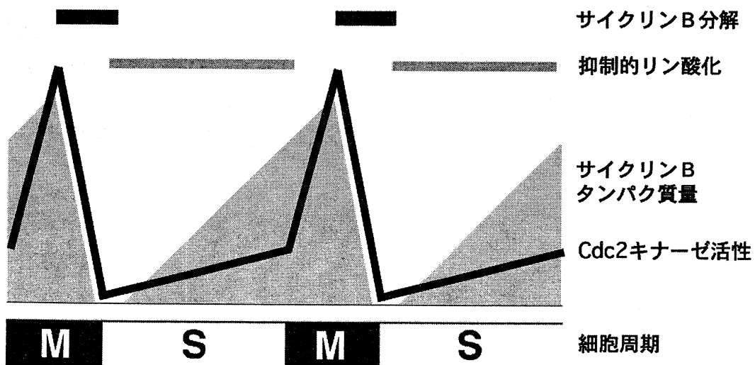
図2 Cdc2キナーゼの活性調節と細胞周期制御
