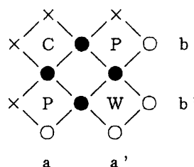
CTM の拡大 (黒丸で和を取る)
