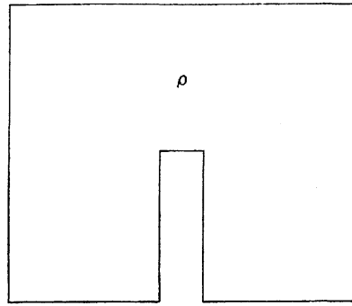
縦に切り開いた密度行列
