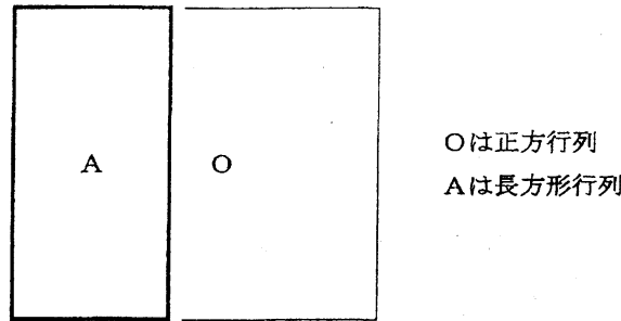
O と A の関係
