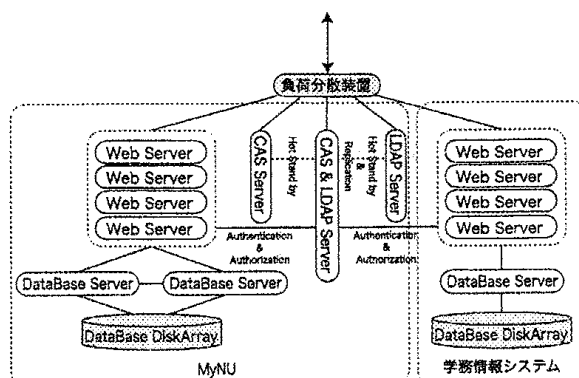
Figure 13: MyNU と学務情報システムのネットワーク構成
