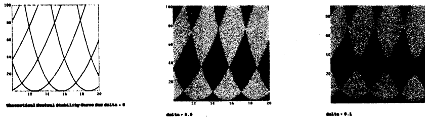
図3: (2)の固定端境界条件での理論的な中立安定曲線(左)と近似計算による固有値分布(中)。明暗の境界が中立安定曲線を表し理論曲線とほぼ一致している。一方、右図は混合型境界条件で \delta = 0.1 とした結果である。1-2モードは交差しているが、2-3モードは擬交差を起こしていることがわかる。
