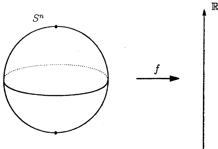
図 1: S^n 上の高さ関数は SGM の典型例
