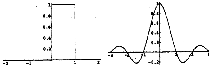
図 1: Haar 関数 \varphi(x) のグラフ (左) と、 |\widehat{\varphi}(t)| = \frac{\sin \pi t}{\pi t} のグラフ (右)
