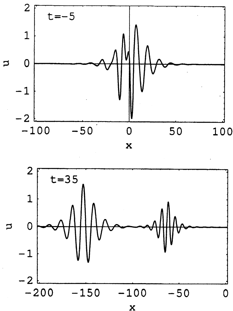
図-3 2個のプリーザーの相互作用; (a) t = -40 , (b) t = -5 , (c) t = 35
