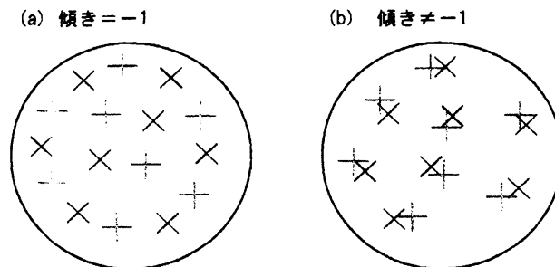
図 12: 正温度側の二つの平衡分布の概念図。2体相関の形から、このような分布であることが予想される。
