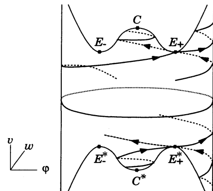
図 2 二等辺 3 体問題の衝突多様体
