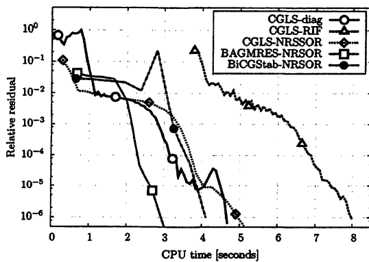
図 4.1: 相対残差 \|A^T r_k\|_2 / \|A^T b\|_2 vs. 計算時間 (LargeRegFile).
