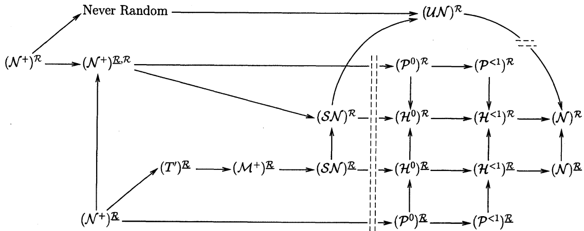
図1 K -トリビアルから非ランダムに至る階層（零加法的集合から零集合に至る階層）：点線内は省略されているが、この間にも途方もなく長い階層が存在する。
