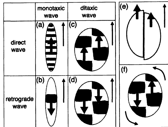
図 2: 腹足類の這行運動時に腹足で観察される筋収縮の波パターンの概略図。(a)monotaxic direct wave. カタツムリやナメクジなどで見られる。(b)monotaxic retrograde wave. アメフラシやヒザラガイ (多板綱) などで見られる。(c)ditaxic direct wave. アワビやカサガイなどで見られる。(d)ditaxic retrograde wave. カサガイの一部やツツノハガイなどで見られる。(e) 左右交互に収縮し動かす。サザエなどで見られる。(f) アワビなどの旋回時の波の様子。
