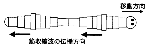
図 1: ミミズの這行運動時の概略図。収縮した体節からは剛毛を出すことが知られている。
