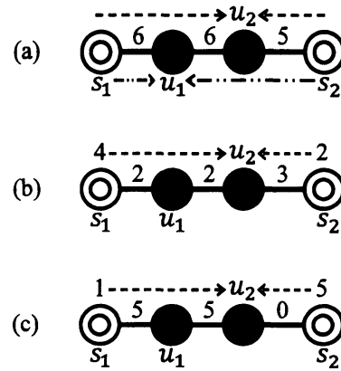
図 1: (a) サーバ割当問題の入力例, (b) 要求 (u_2, 6) を満たすサーバ割当 \mathbf{a} , (c) 要求 (u_2, 6) を満たす最適なサーバ割当 \mathbf{a}^* .
