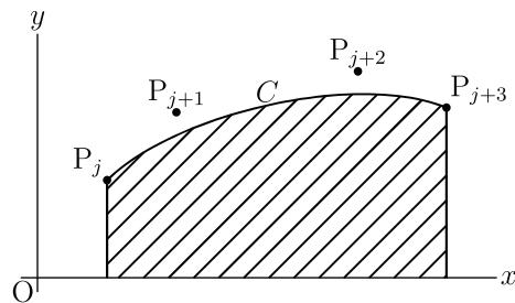
図 12 Bézier 曲線の積分
