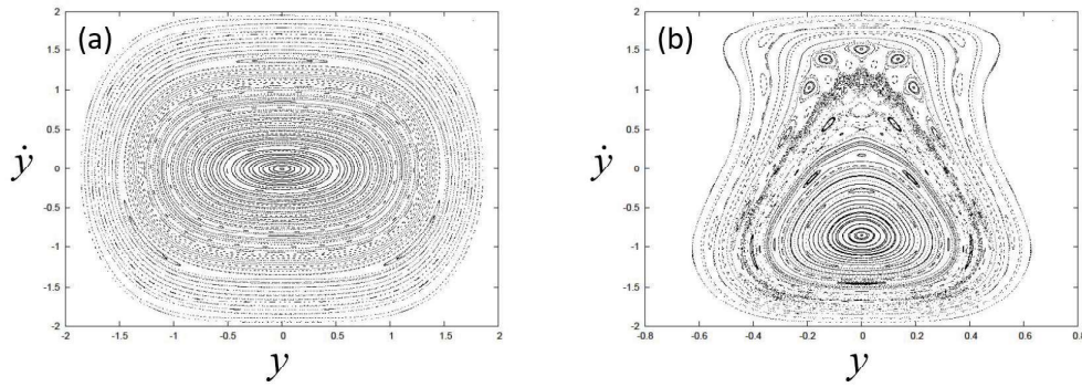
図 1: 簡約力学系 (43), (44) のポアンカレ断面: \omega_k = \omega_{3k} = 0 , (a) k = 0.67\pi , (b) k = 0.8\pi .
