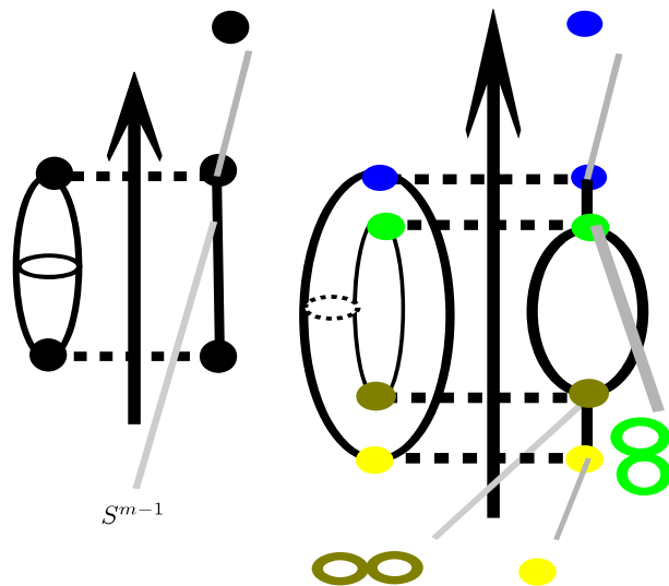
Figure 1: 次元 2 以上の単位球面の自然な高さを考えて得られる Morse 関数と Reeb グラフ(左). \mathbb{R}^3 に自然な形で埋め込まれたトーラス( S^1 \times S^1 )に対し自然な高さを考えて得られる Morse 関数と Reeb グラフ(右). グラフの点を指し示す線のある点や円周等の図形や単位球面 " S^{m-1} "の表記は, その点の q_f で考えた逆像を示す: なお右のグラフで辺(の内部)の各点の逆像は円周.
