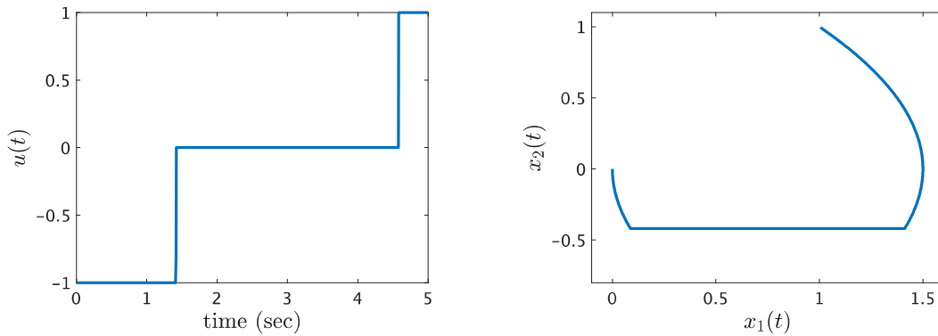
図 2 左図は提案したアルゴリズム 3.1 を適用して得られた制御 u(t) のグラフ。右図は、左図の制御 u(t) に対応する状態 \{\boldsymbol{x}(t) = (x_1(t) \ x_2(t))^T \ (0 \leq t \leq 5)\} の軌跡。初期状態 \boldsymbol{x}(0) = (1 \ 1)^T から \boldsymbol{x}(5) = (0 \ 0)^T に遷移しているのがわかる。
