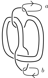
Figure 7.5: The map \pi_1(S^3 \setminus K) \rightarrow \langle a, b \mid a^{-1}ba^{-1}bab^{-1} \rangle
