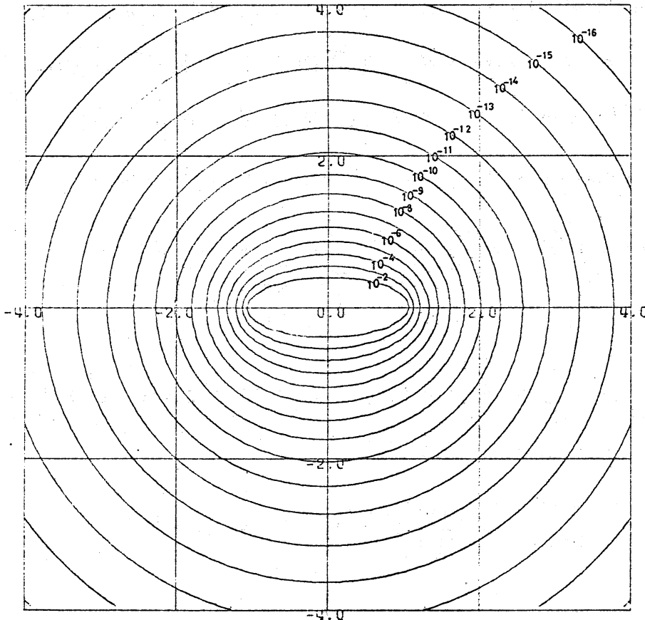
★ 2 図 Legendre-Gauss 公式 ( n=8 ) の |\Psi(z)| の等高線図
