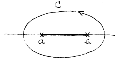
※ 1 回 (1-4) の積分路 C
