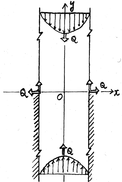
図 2 点 (\pm 1, 0) に点吸い込みと点すべりのあるときの管路の流れ (4.3)
