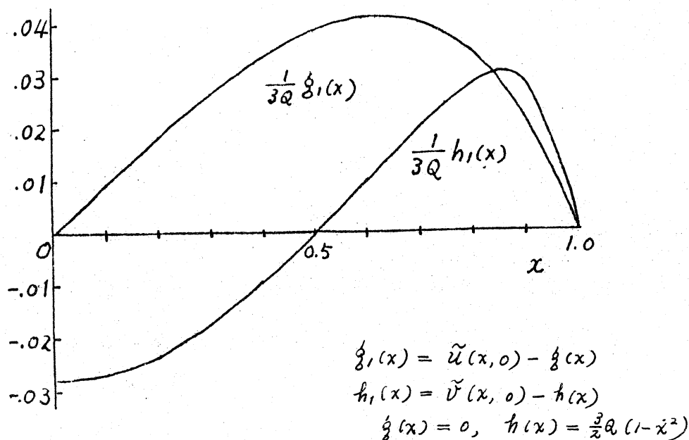
図 3. 出口においてはじめて発達したポアズイユの流速分布からのずれ。
