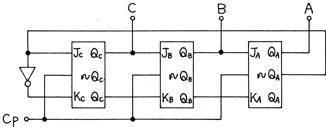
図8 9進ダブル・サイクリング計数器
