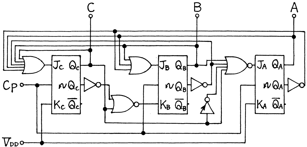
図5 3値減算型JK-FFを用いた 10進減算計数器
