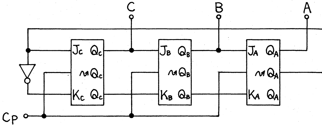
図7 9進サイクリング計数器
