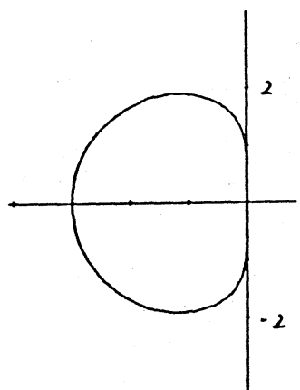
图11. 3段4次Adams-Moulton法
