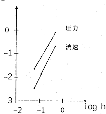
図 8 表面張力を考慮しないテスト問題の誤差
