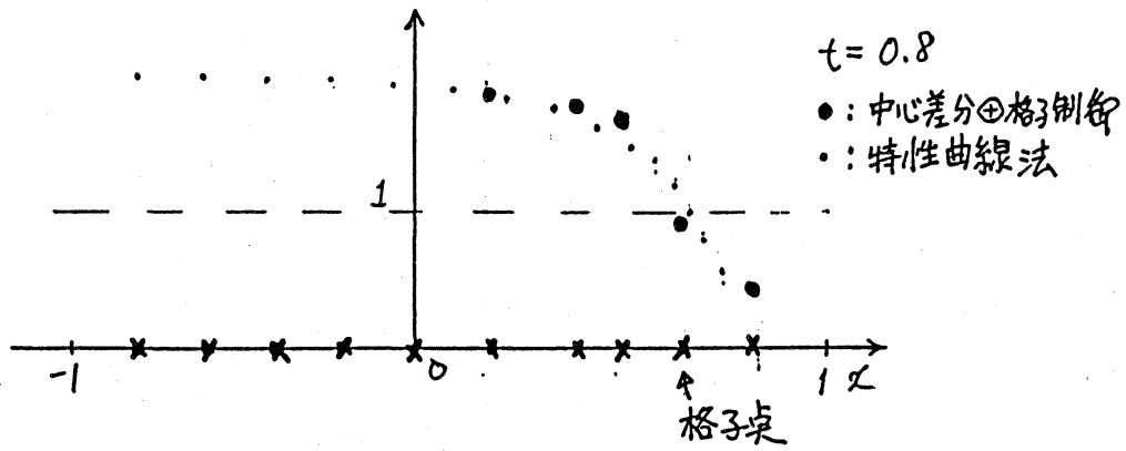
図2 パーガーズ方程式への応用
