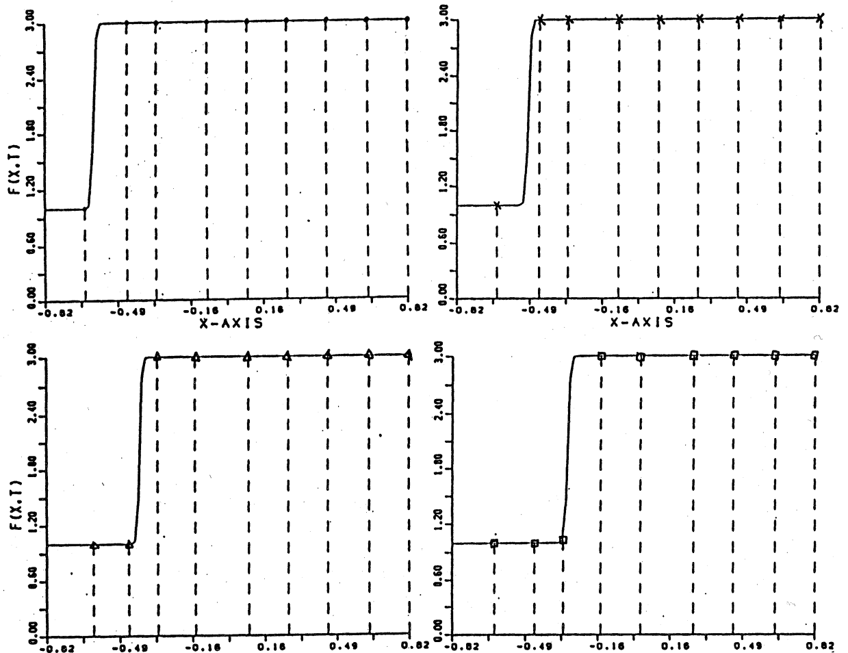
図1 ファジィ推論による格子の移動
