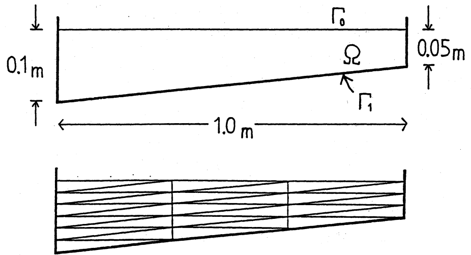
図1 静止水域 \Omega とそのフリードックス・ケラー型三角形分割 ( I = 3 の場合)
