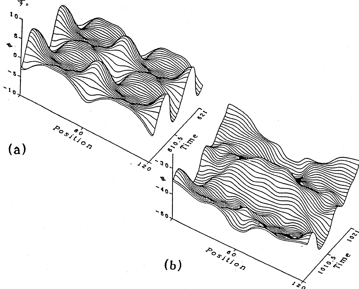
図2. SG方程式: \phi_{tt} - \phi_{xx} + \sin \phi = \gamma \sin \omega t - \varepsilon \phi_t の数値解 (\varepsilon = 0.2, \omega = 0.6) (a) 周期的発展 ( \gamma = 0.8 ) (b) カオス的発展 ( \gamma = 1.0 )
