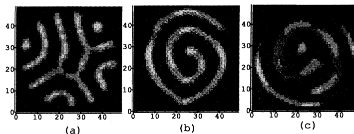
図 8: 3次元回転系
