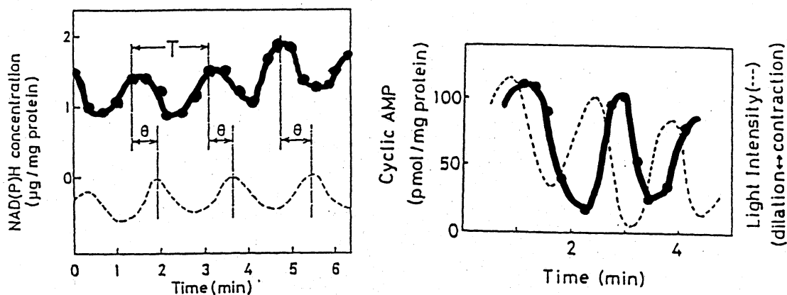
図 3 : 移動中の粘菌の進行端における細胞内 NADH 濃度 (左) とサイクリック AMP 濃度 (右) の振動。 波線は、原形質の厚み振動を示す。
