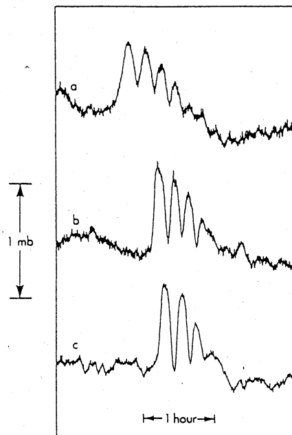
図 6: 微気圧計による観測記録 [Christie(1989)] 観測地点: Edward River (ER) 各々の開始時刻、発生源の方位角、伝播速度は (a) 1983年9月15日 21:52 EST、28 deg.、5.9m/s (b) 1983年9月18日 21:20 EST、31 deg.、6.3m/s (c) 1983年9月24日 21:17 EST、35 deg.、7.2m/s
