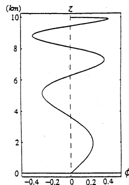
図 16: c_0 = 18.7m/s に対応する鉛直構造関数 \phi(z)
