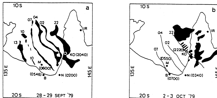
図 5: GMS 「ひまわり」の赤外面像によるモーニンググローリーの雲の動き [Clarke et al.(1981)] (a) 1979 年 9 月 28 日 - 29 日 (b) 1979 年 10 月 2 日 - 3 日 観測点の数字は気圧ジャンプの通過時刻
