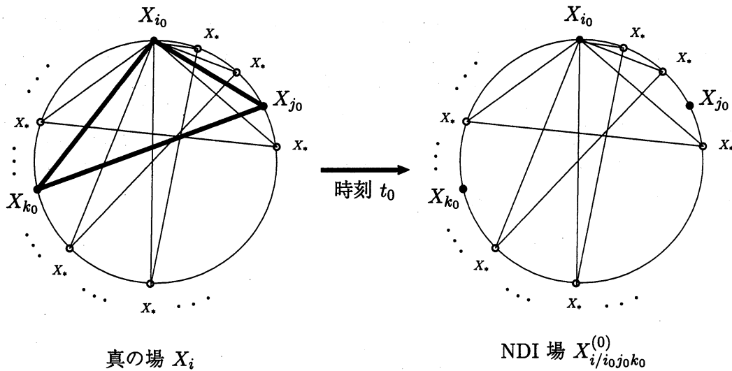
図 2: 直接相互作用分解 時刻 t_0 において特定の 3つのモード X_{i_0} , X_{j_0} , X_{k_0} の間の直接相互作用を人為的に抜き去ることによって作られるのが NDI 場 X_{i/i_0j_0k_0}^{(0)} である. この 1つの直接相互作用を消去することにより, これら 3つのモード間には, ひとつも直接相互作用がないことに注意されたい. これは系のもつ『弱い非線形結合』の性質による.
