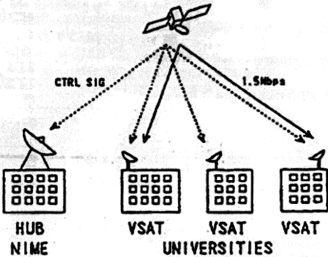
图 1: SCS 構成図
