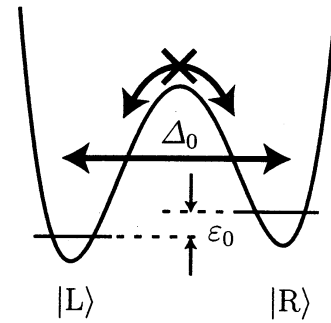
図 3: 二準位系.
