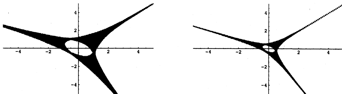
図 6: W(x, y) = x + y + \frac{1}{xy} + 3 = 0 の (x, y) \mapsto (\log_t |x|, \log_t |y|) による像 (左が t = 3 、右が t = 10 ).
