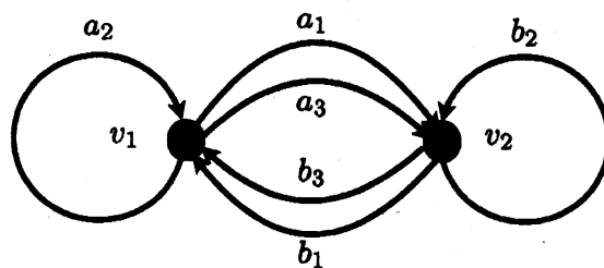
図 32: 図 31 から籠だけを取り出したもの
