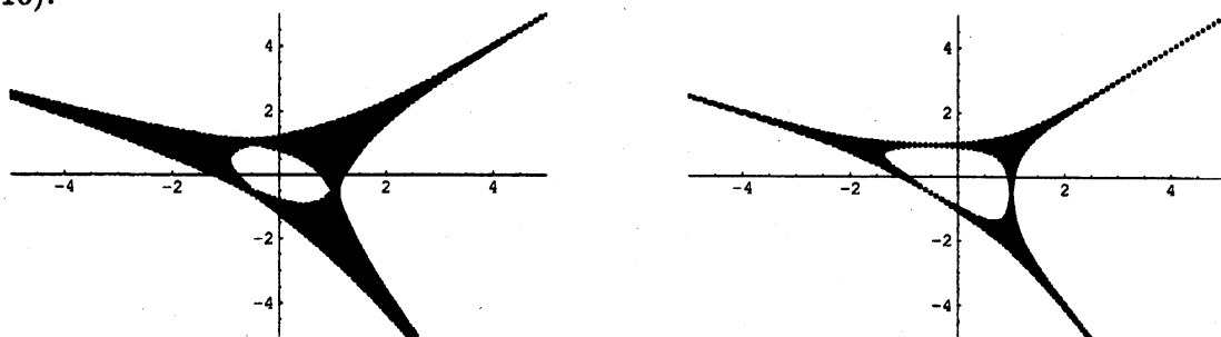
図 7: W(x, y) = x + y + \frac{1}{xy} + t = 0 の (x, y) \mapsto (\log_t |x|, \log_t |y|) による像 (左が t = 3 、右が t = 10 ).
