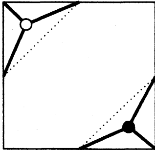
図 23: \Delta_1 に対応する 2 色グラフ
