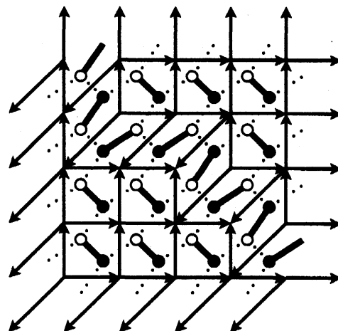
図 46: ダイマー配置と部分箭の関係
