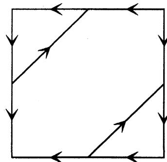
図 12: W_{\Delta_1}^{-1}(0) の葉の漸近境界
