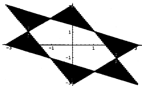
図 8: W(x, y) = x + y + \frac{1}{xy} の零点の藻
