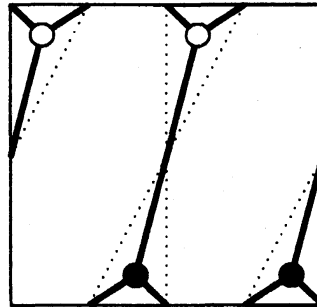
図 24: \Delta_2 に対応する 2 色グラフ
