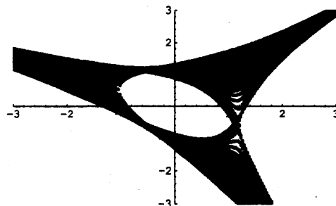
図 2: W(x, y) = x + y + \frac{1}{xy} の零点のアメーバ 図 3: W(x, y) = x + y + \frac{1}{xy} + 3 の零点のアメーバ
