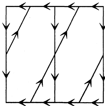
図 16: W_{\Delta_2}^{-1}(0) の藻の漸近境界
