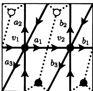
図 31: \Delta_2 に対応する籠
