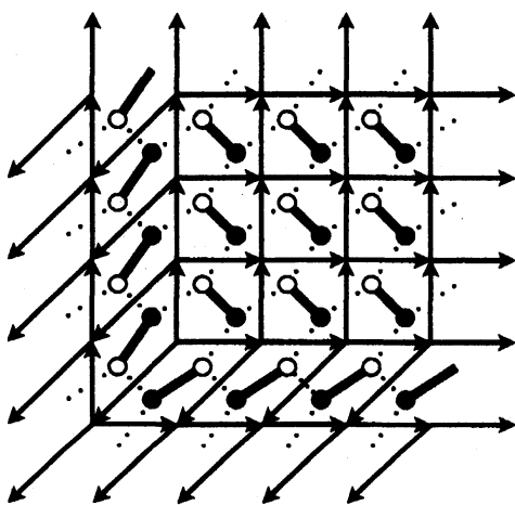
図 47: 「空の」ダイマー配置
