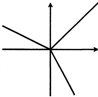
図 4: W(x, y) = x + y + \frac{1}{xy} + 3 に対する W^{-1}(0) の非アルキメデスのアメーバ
