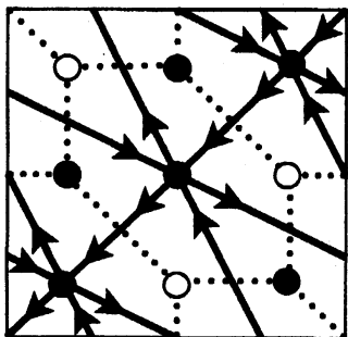
図 33: \Delta_3 に対応する籠
