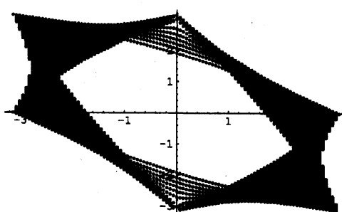
図 9: W(x, y) = x + y + \frac{1}{xy} + 3 の零点の藻
