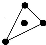
図 1: Newton 多角形
