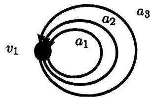
図 30: 図 29 から籠だけを取り出したもの
