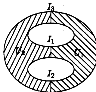
図 12: W_{\Delta_1}^{-1}(0) の葉の漸近境界
