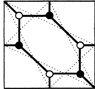
図 25: \Delta_3 に対応する 2 色グラフ
