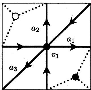
図 29: \Delta_1 に対応する籠
