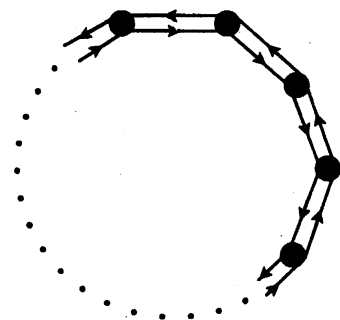
図 35: 1 次元の時の籠
