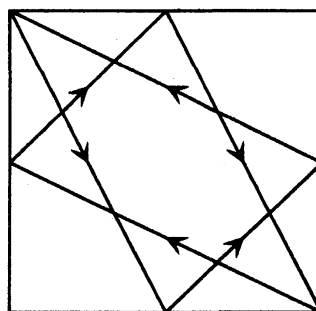
図 20: W_{\Delta_3}^{-1}(0) の藻の漸近境界
