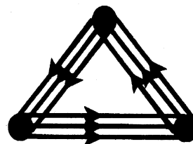
図 34: 図 33 から籠だけを取り出したもの
