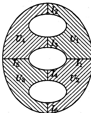
図 16: W_{\Delta_2}^{-1}(0) の藻の漸近境界
