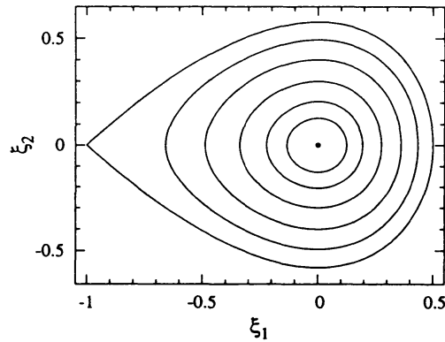
図 2. 式 (10) の \xi 平面上の周期軌道族 \xi^k(t)
