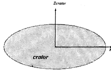
図 15: クレーターの座標軸
