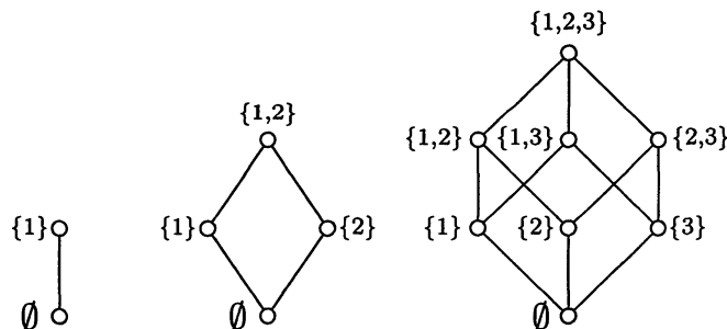
図 1. Boolean 代数
