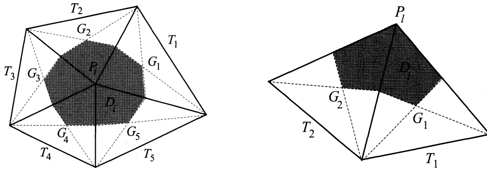
(a) 内部節点 $P_i$ の重心領域 $D_i$ (b) 境界節点 $P_l$ の重心領域 $D_l$
