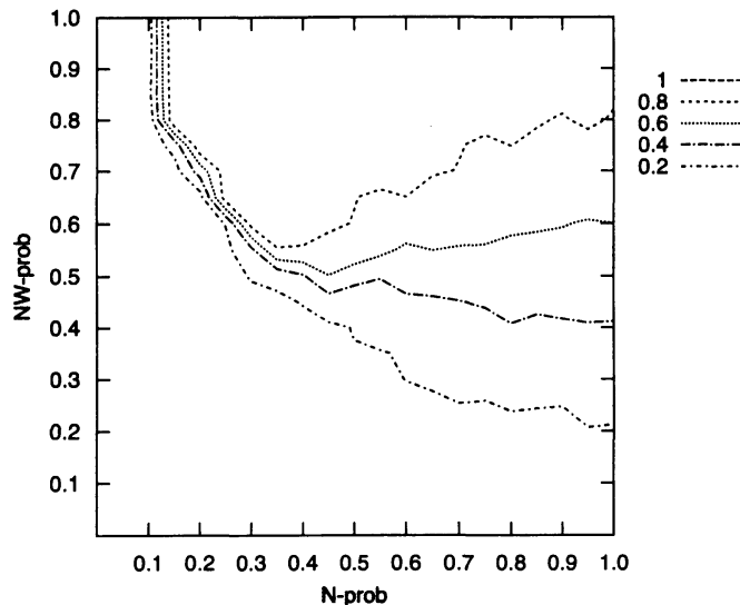
Figure 1 N \cdot \text{prob} 、 NW \cdot \text{prob} と私語率の関係（シミュレーションによる）
