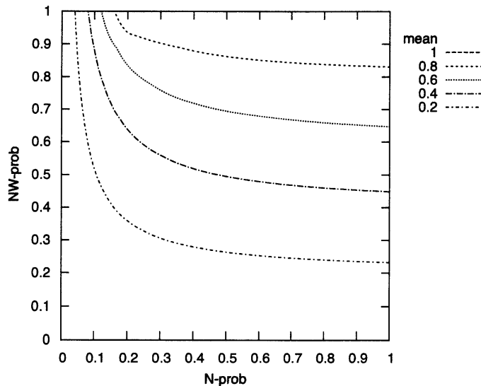
Figure 2 N-prob、NW-prob と私語率の関係 (平行場近似による)
